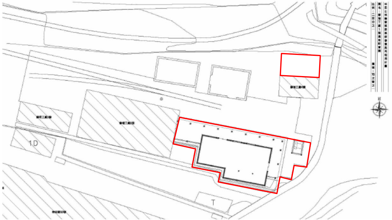
圖2：林田山林业文化園區-木工室(修理工廠一館)暨周邊租賃土地範圍套繪圖 (上方紅框作為木料暫時儲放區/下方紅框為工作和展售區)
