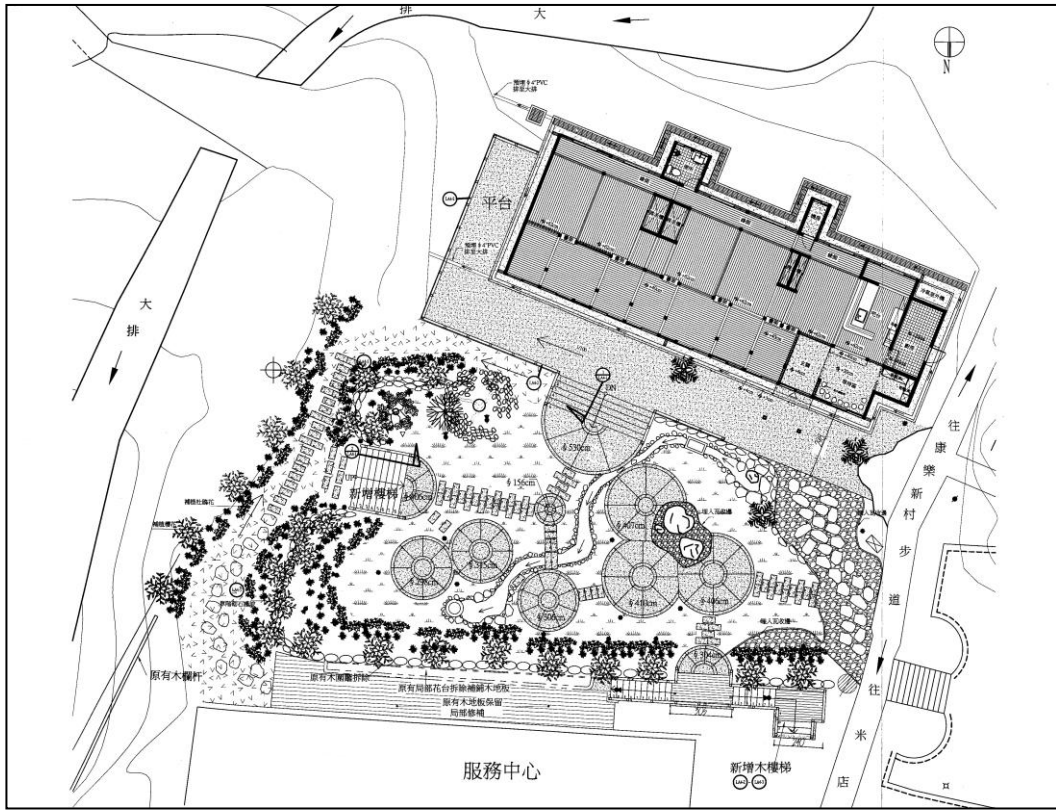
圖 3. 林田山林業文化園區服務中心二館平面圖
