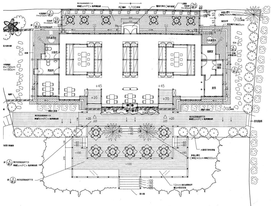
圖 2. 林田山林業文化園區服務中心一館平面圖
