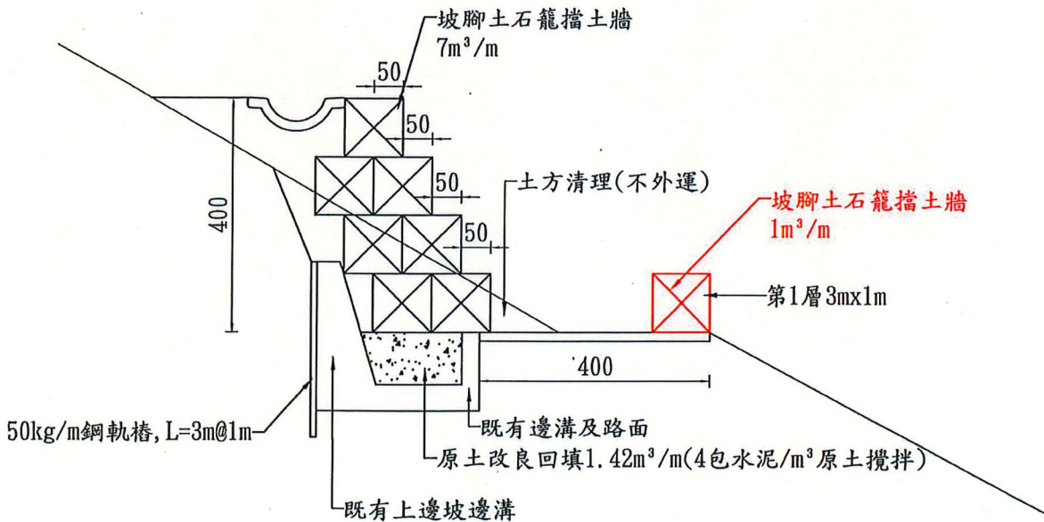
坡腳處理斷面圖(竣工修正)
