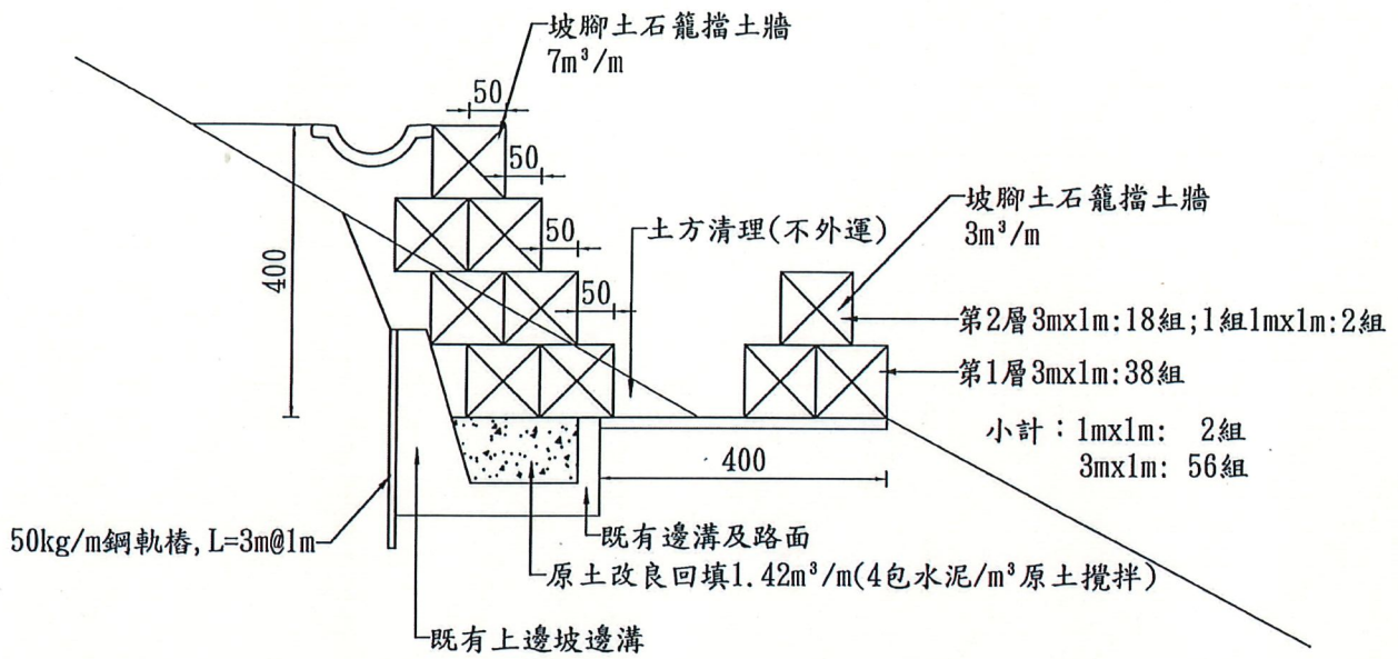
坡腳處理斷面圖(原契約)
